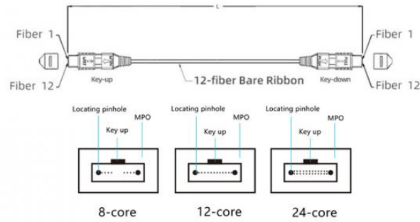
MPO/MTP 12Core
